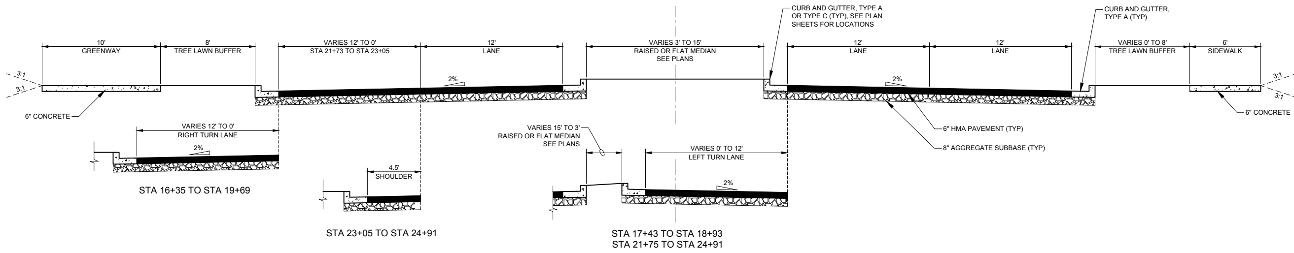
STA 16+35 TO STA 24+91
